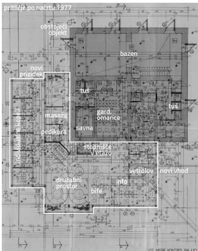
Načrti preureditve bazenskega objekta za pridobitev gradbenega dovoljenja iz leta 1977. 102
