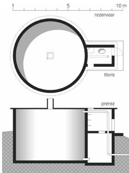
Vodovodni rezervoar v Topolšici, izmera in risba R. Poles, 2022.
