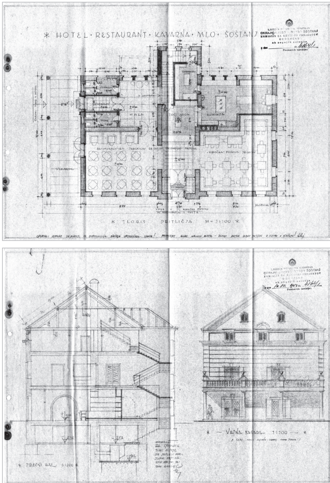
Del načrtov za prenovo hotela MLO Šoštanj, datirani so z 10. 10. 1952, še preden je hotel postal družbena lastnina. 101
