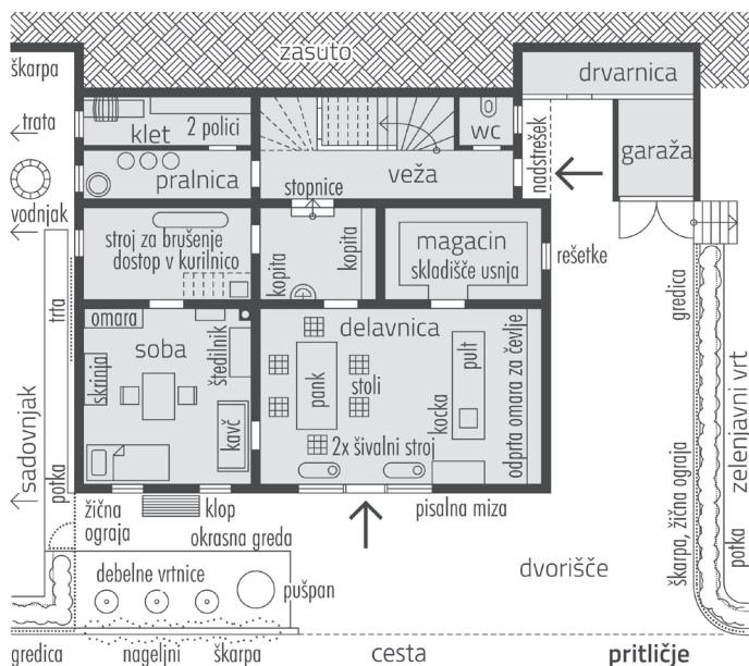
Pritliče naše hiše v Šoštanju.
